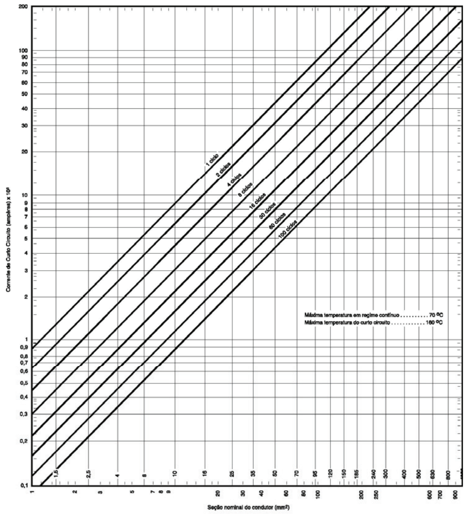
Figura 9 – Corrente máxima de curto circuito para fios e cabos isolados com PVC
